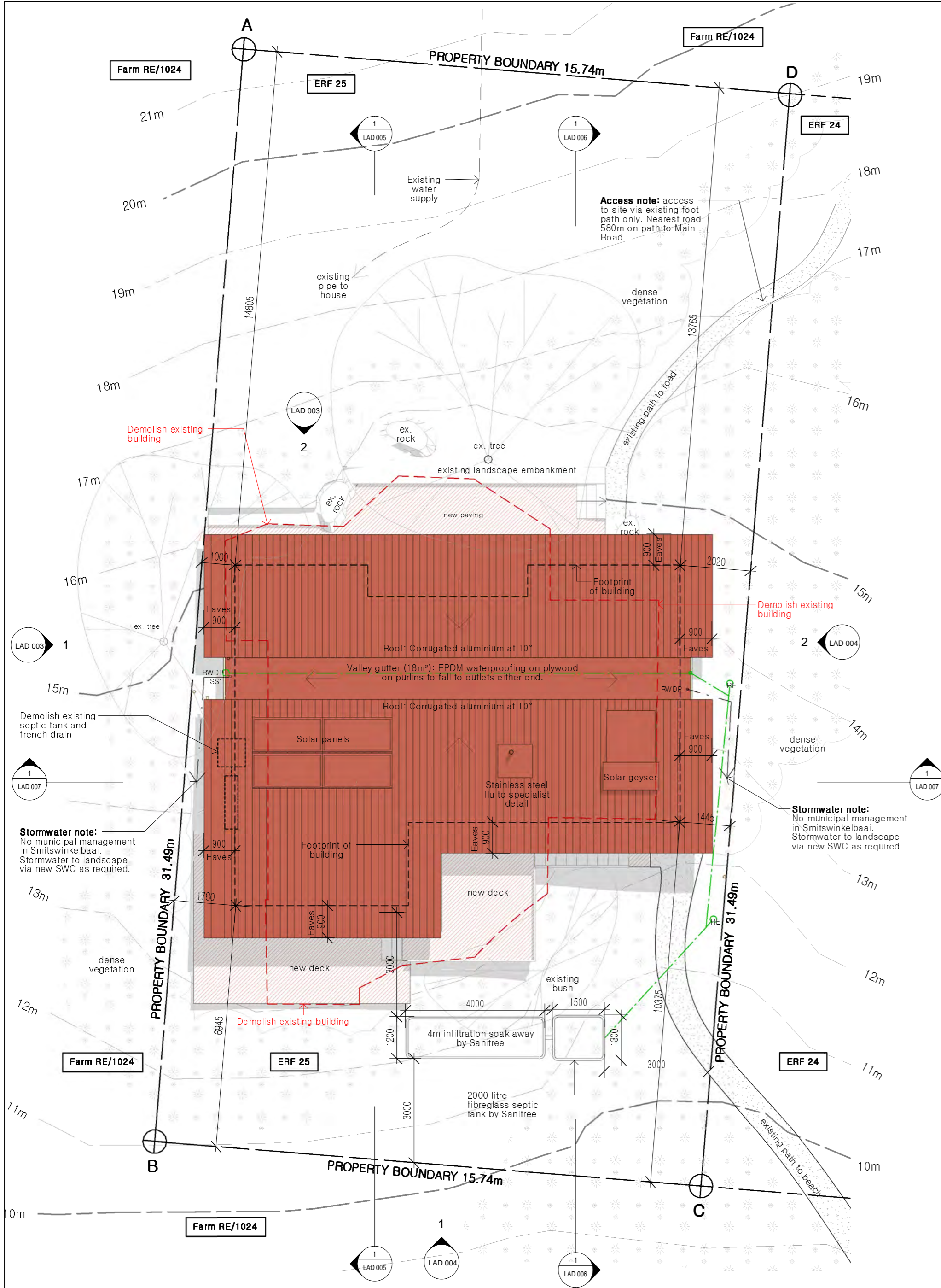
1 Site plan 1 : 100
